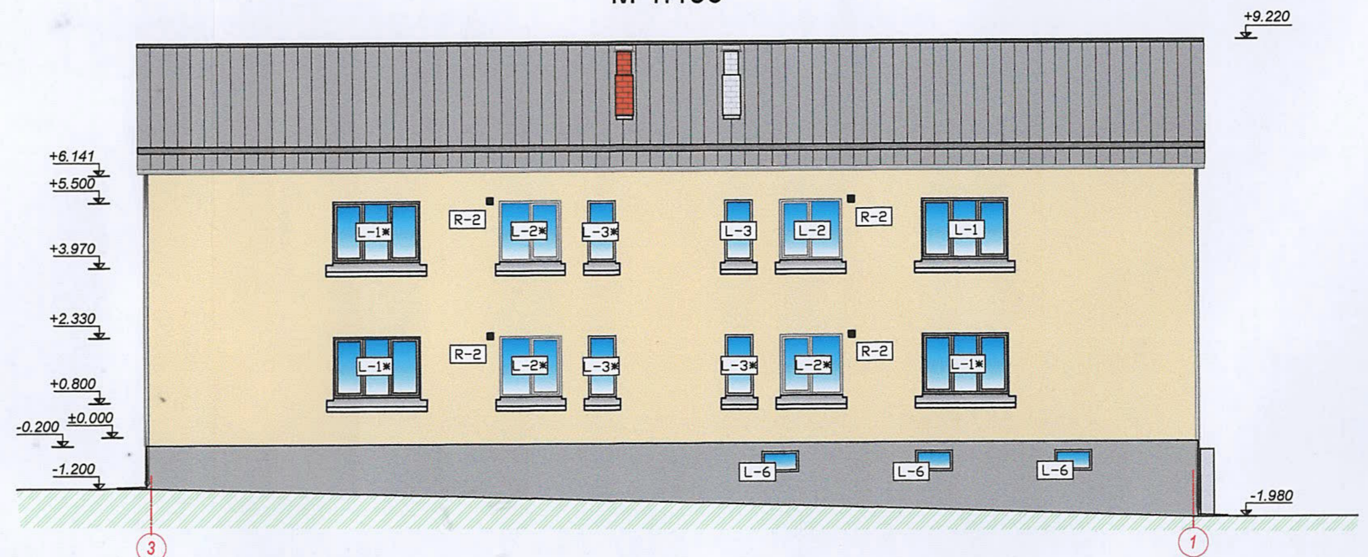
Fasāde asīs 3-1 M 1:150
