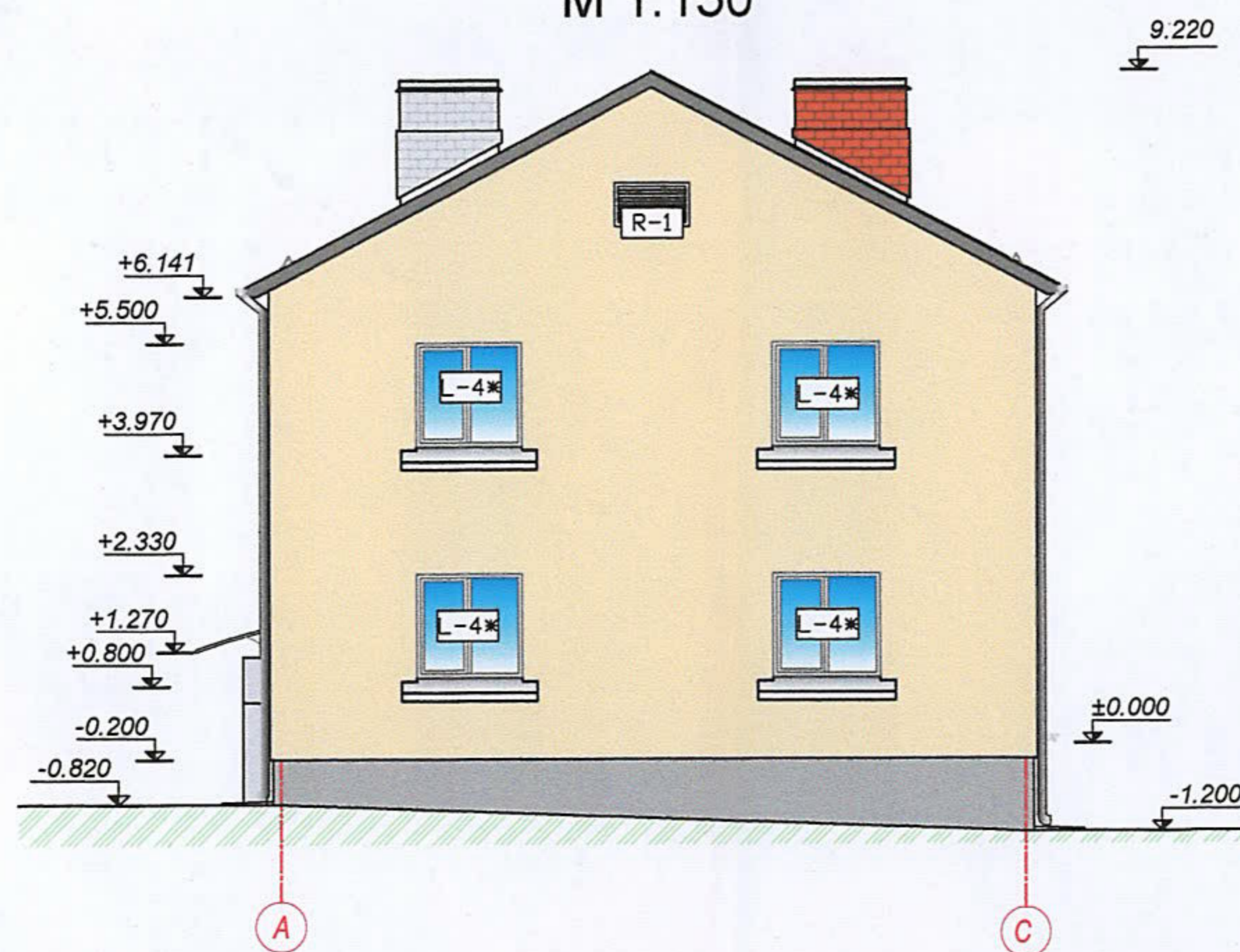
Fasāde asīs A-C M 1:150
