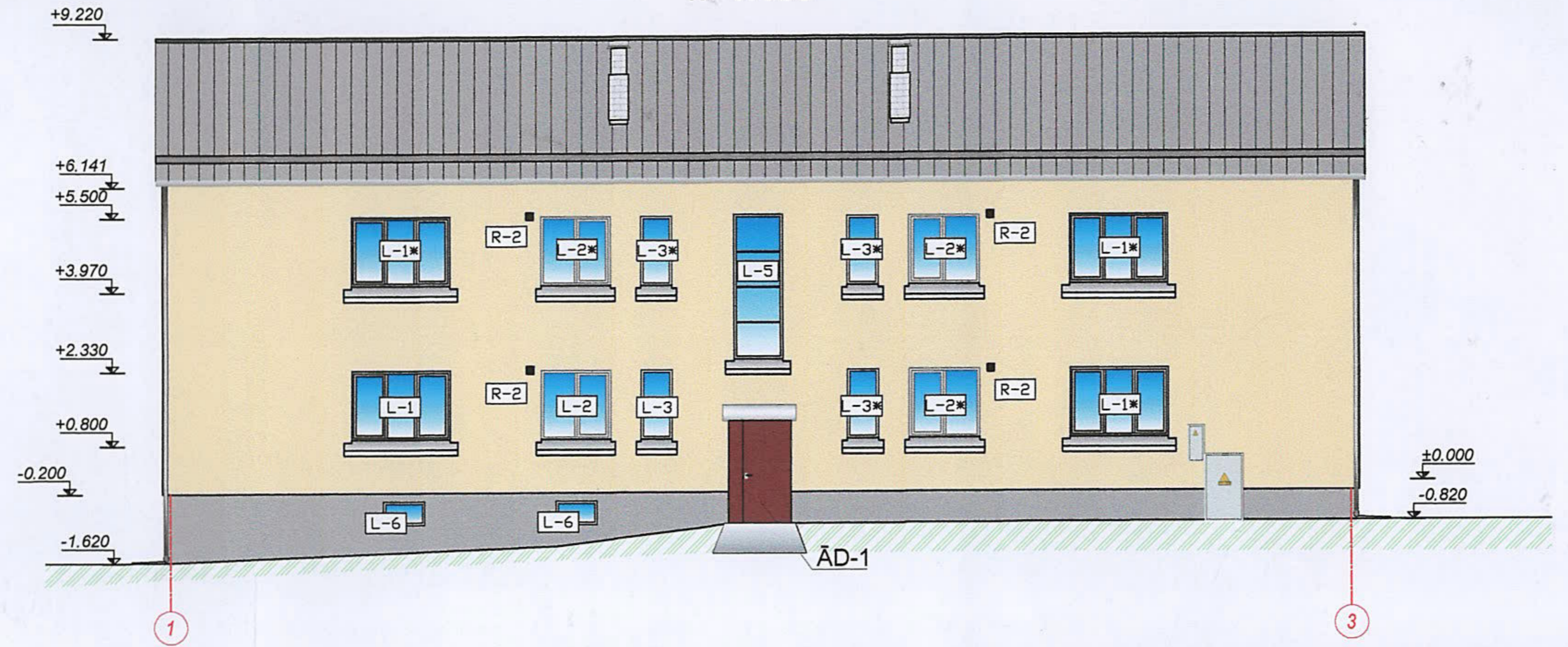
Fasāde asīs 1-3 M 1:150
