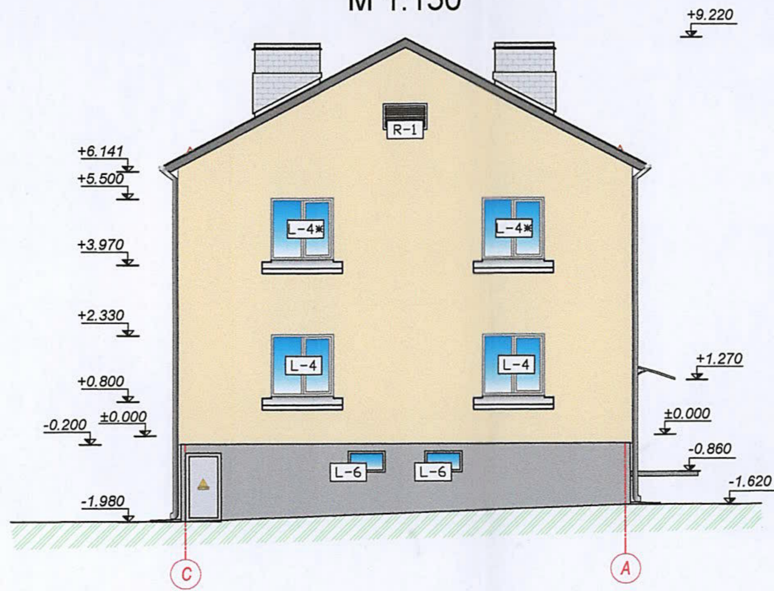
Fasāde asīs C-A M 1:150
